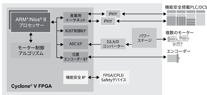
図 5-1：モーター制御
